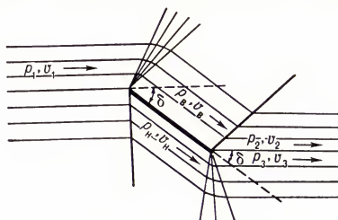
Рис. 3. Схема сверхзвукового обтекания пластинки: v_n > v_1 , p_n < p_1 ; v_2 < v_n , p_2 > p_n ; v_n < v_1 , p_n > v_1 ; v_3 > v_n , p_3 < p_n .
